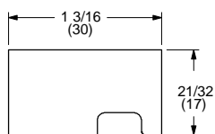
W7084 – Side Blind Stop, Picture
